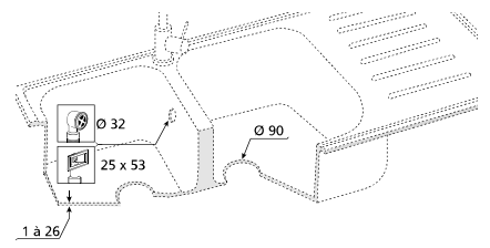
Ø 90 MM SIMPLES PAREDE : INOX, ACRILICO, CERÂMICA
